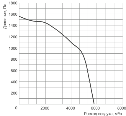
SDT 70-40/31.2D-2,2
