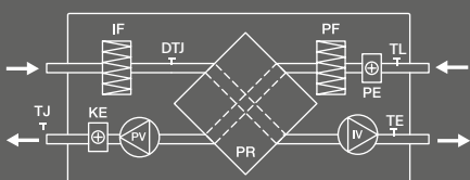
HPE 450, HPE 800
