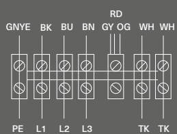
Схема 2 (400 В, 3 ф, 50 Гц.)
