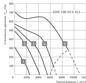
Схема 4 (λ — 400 В, 3 ф.)
