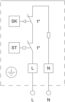
Схема 1 (230 В, 1 ф.)
