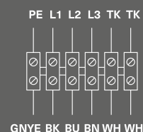
Схема 5 (λ — 400 В, 3 ф.)
