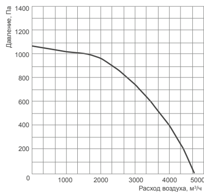
SDT 60-35/31.2D-1,5
