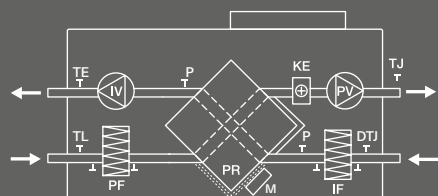
CPE 1000, CPE 1500
