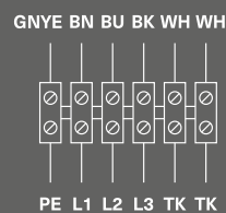
Схема 3 (400 В, 3 ф, 50 Гц.)
