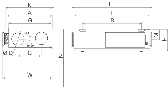
CPE 1500
