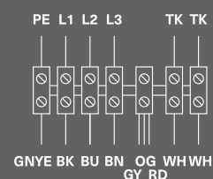
Схема 4 (λ — 400 В, 3 ф.)
