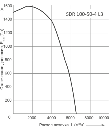
Схема 2 (400 В, 3 ф, 50 Гц.)
